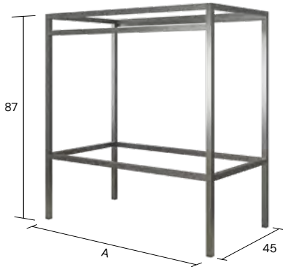
Floor standing Sur pied A pavimento
